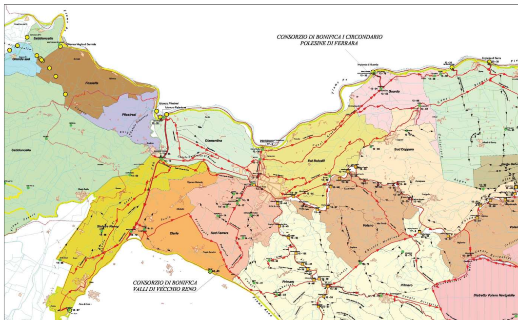
Fig. 22 - Rete e distretti irrigui
