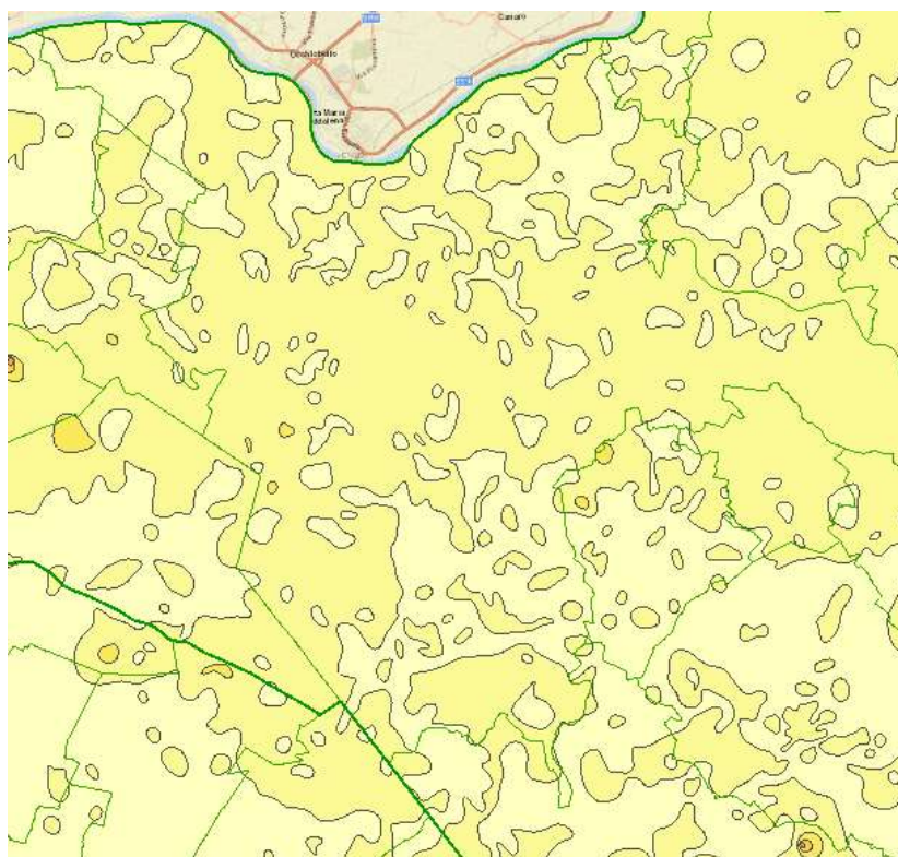
Fig. 12 - Subsidenza – periodo 2016-2021
