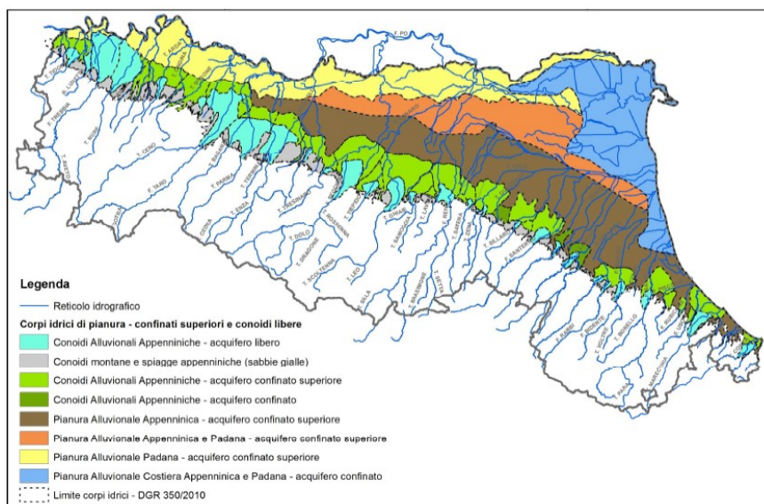
Fig. 42 - Corpi idrici sotterranei di pianura liberi e confinati superiori
