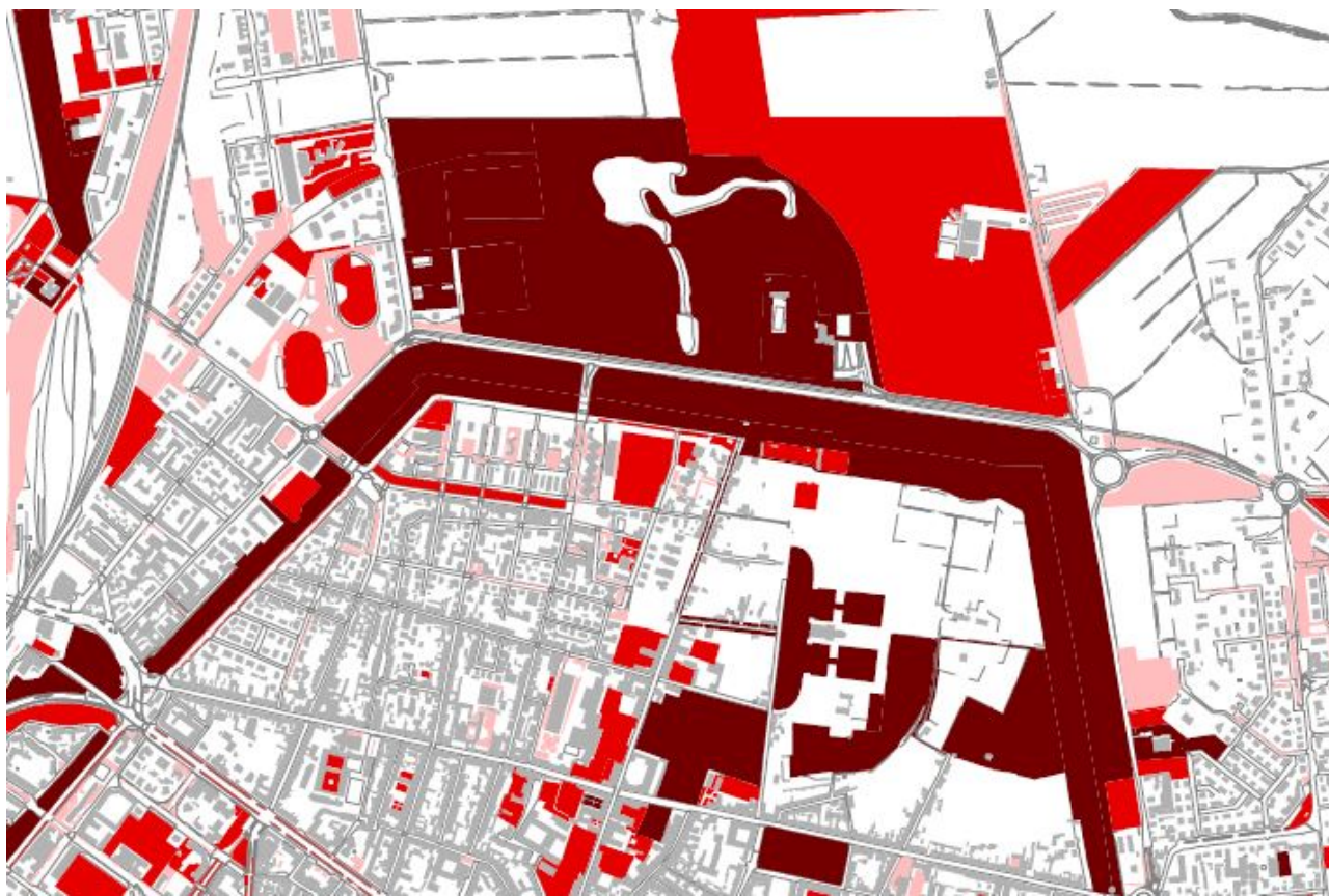
Fig. 19 – Il livello di erogazione dei servizi ecosistemici culturali: alto, medio, basso (estratto esemplificativo dell'elaborato QC.5.3.4b SERVIZI ECOSISTEMICI CULTURALI)
