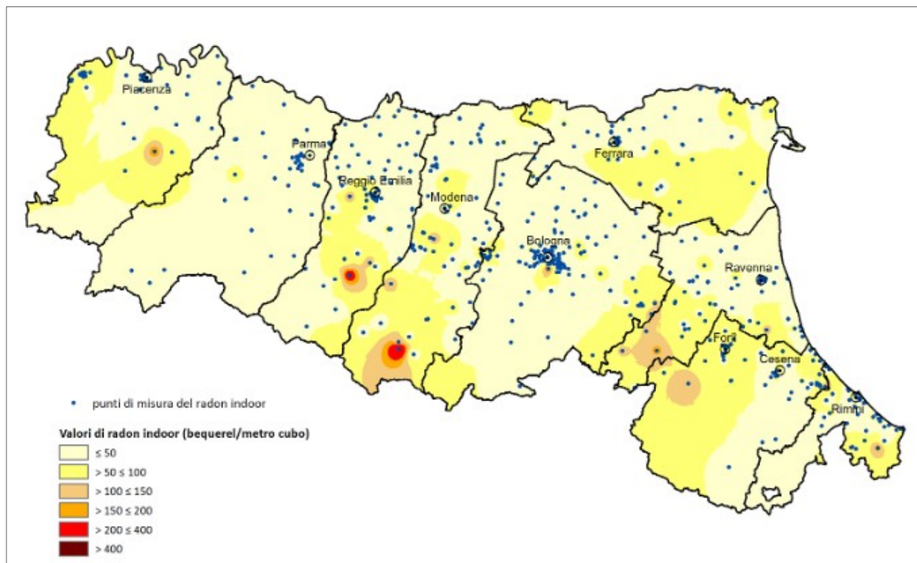
Fig. 57 - Rappresentazione cartografica dei punti di misura del radon indoor relativi alle indagini condotte nelle abitazioni e nelle scuole e curve di isolivello delle concentrazioni
