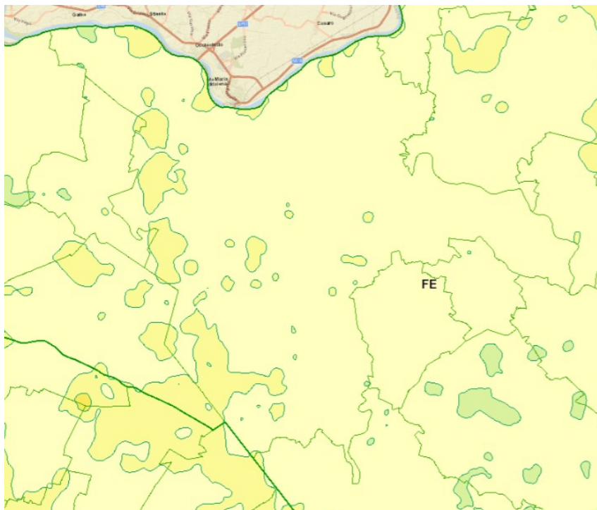
Fig. 10 - Subsidenza – periodo 2006-2011
