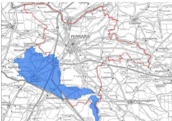
Fig. 50 - Aree allagate a seguito dell'alluvione del 1951
