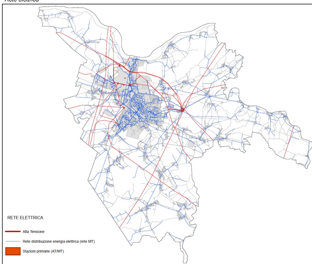
Fig. 54 – Rete elettrica
