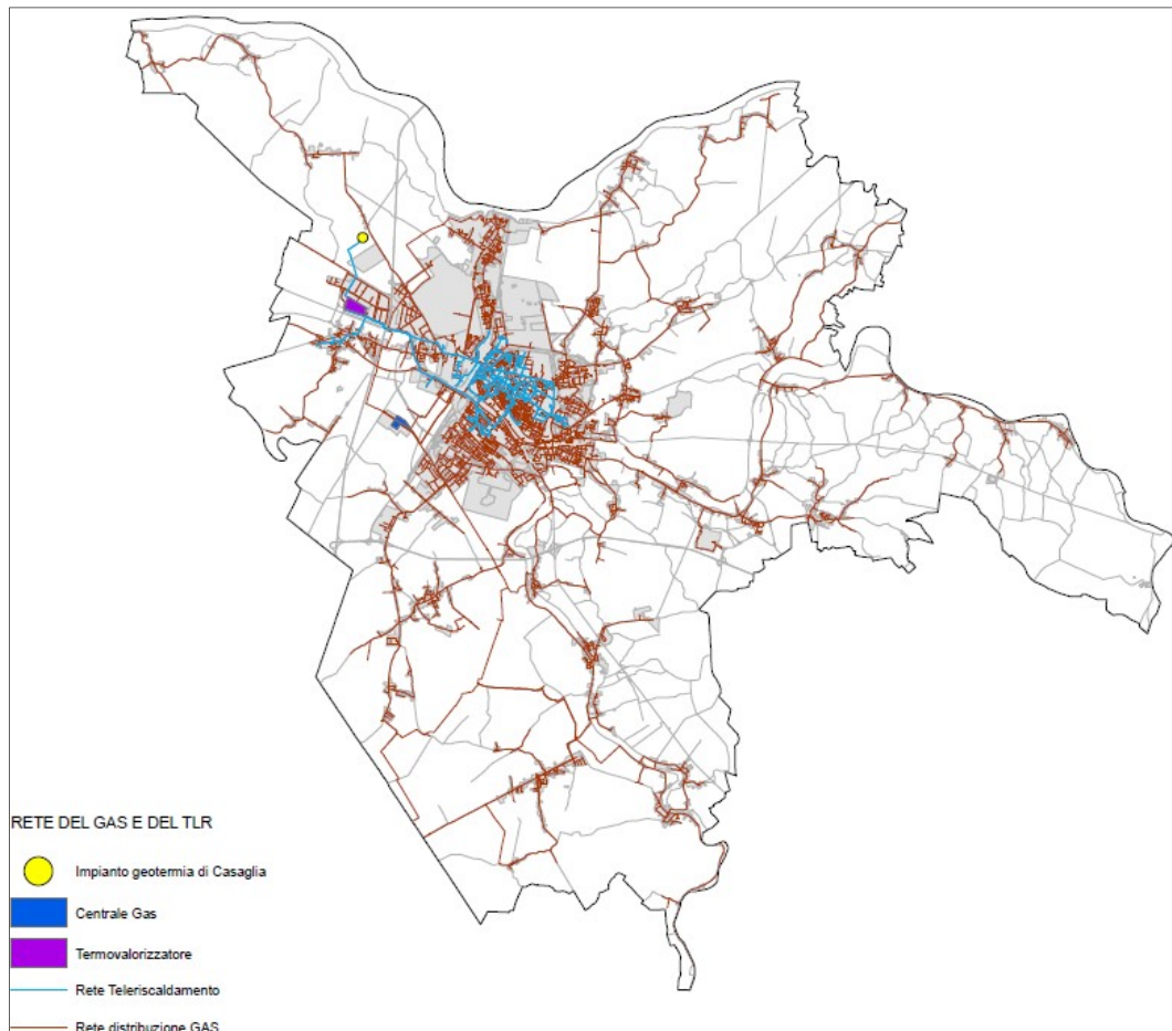
Fig. 55 – Rete del Gas e del Teleriscaldamento
