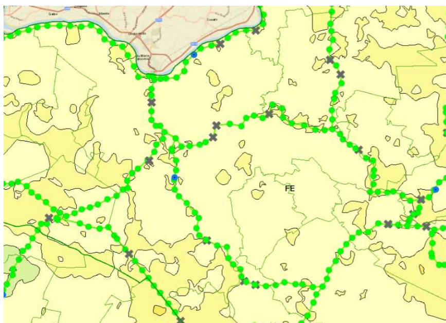
Fig. 11 - Subsidenza – periodo 2011-2016
