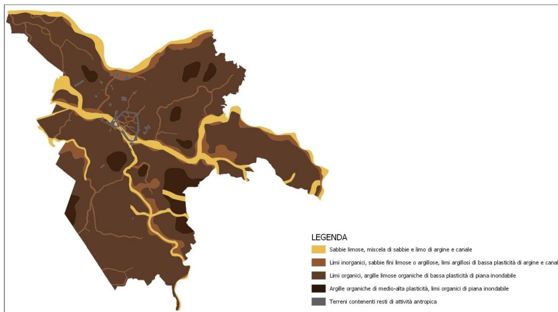
Fig. 6 - Carta geologico-tecnica del Comune di Ferrara (elaborazione 2020)
