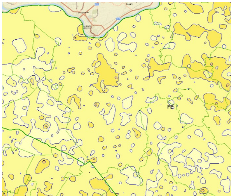
Fig. 9 - Subsidenza – periodo 2002-2006
