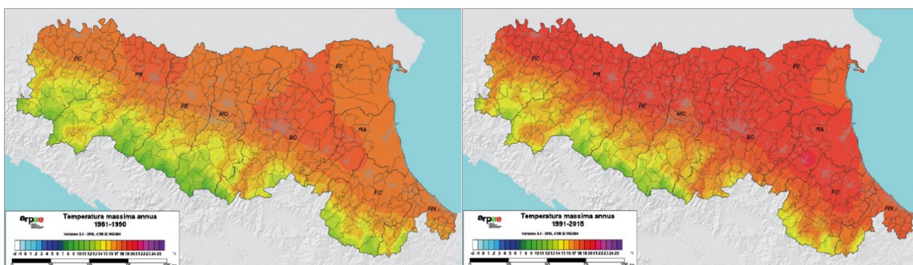
Fig. 27 - Temperature medie massime dell'Emilia Romagna nel periodo 1961-1990 e 1991-2015; fonte ARPAE 2017
