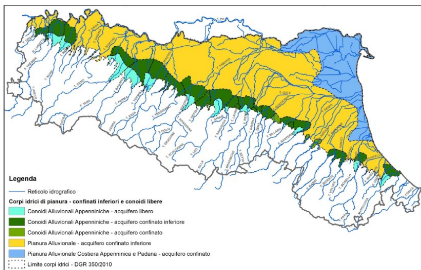
Fig. 43 - Corpi idrici sotterranei di pianura confinati inferiori
