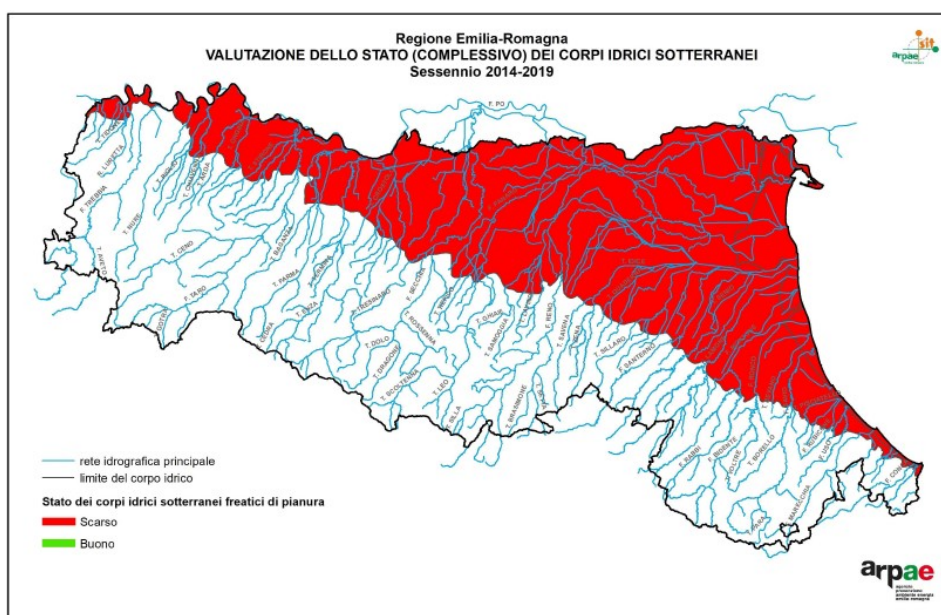
Fig. 46 - Valutazione stato complessivo dei corpi idrici freatici di pianura (2014-2019)
